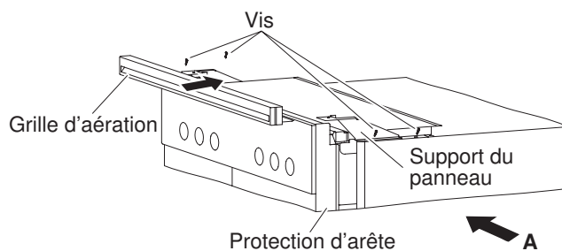
Vue A Four 55-381, 60-381
