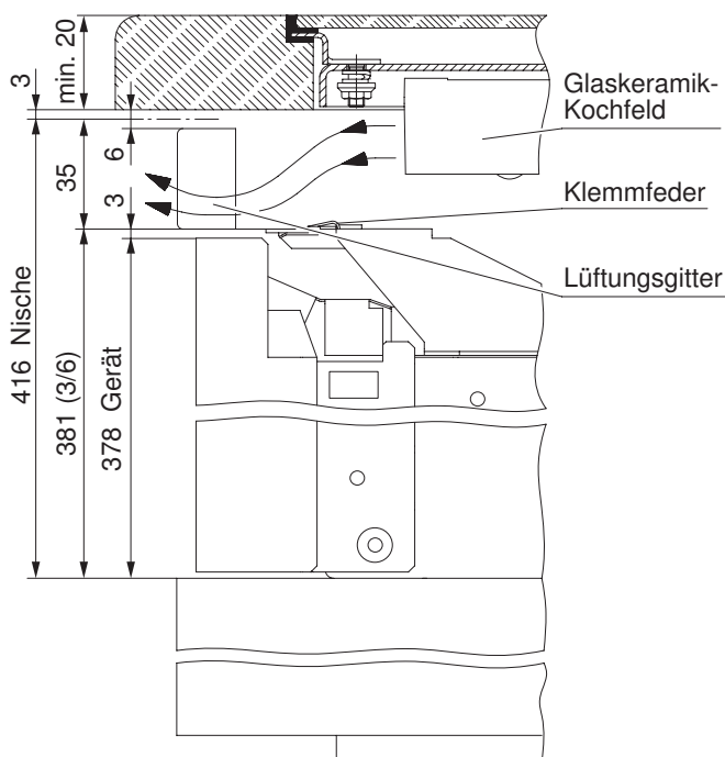
Ansicht A Backofen 55-381, 60-381
