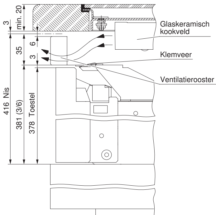
Aanzicht A Bakoven 55-381, 60-381
