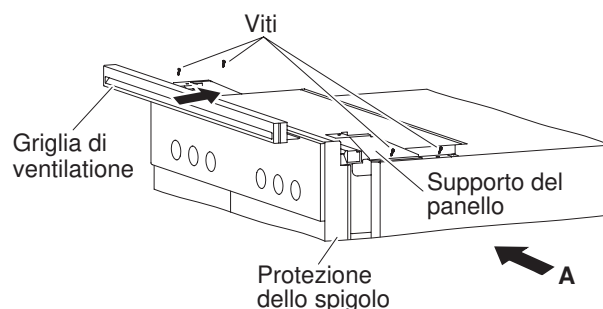
Veduta A Forno 55-381, 60-381
