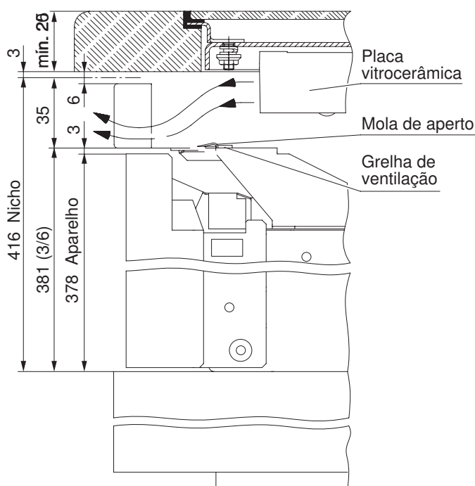
Vista A Forno 55-381, 60-381
