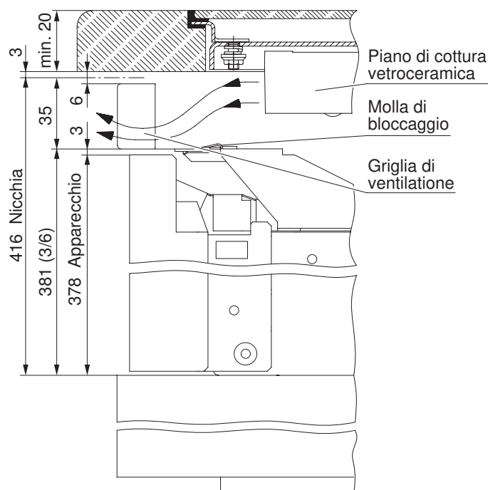
Veduta A Forno 55-381, 60-381
