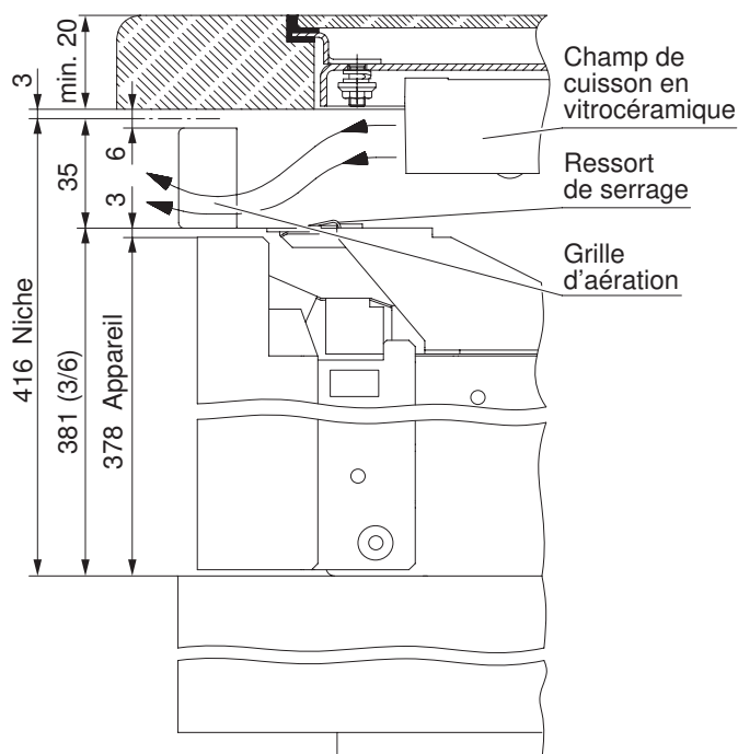
Vue A Four 55-381, 60-381
