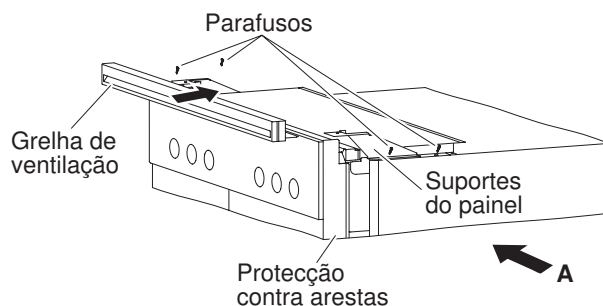
Vista A Forno 55-381, 60-381
