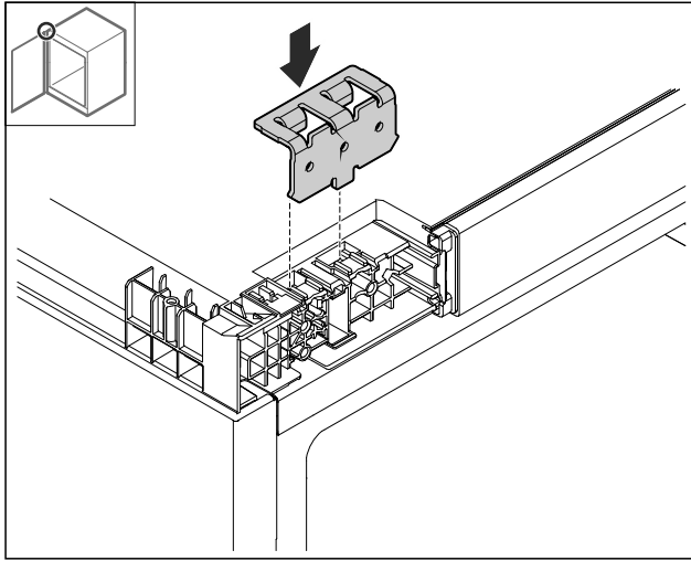
Fig. 23 ► Winkel einsetzen.
