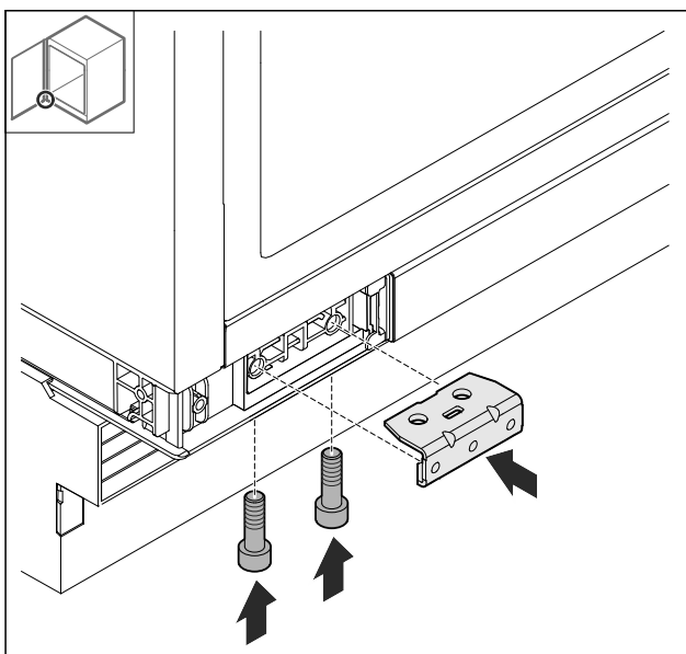
Fig. 25 ► Winkel montieren.
