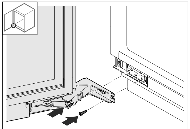
Fig. 27 ► Tür unten anschrauben.
