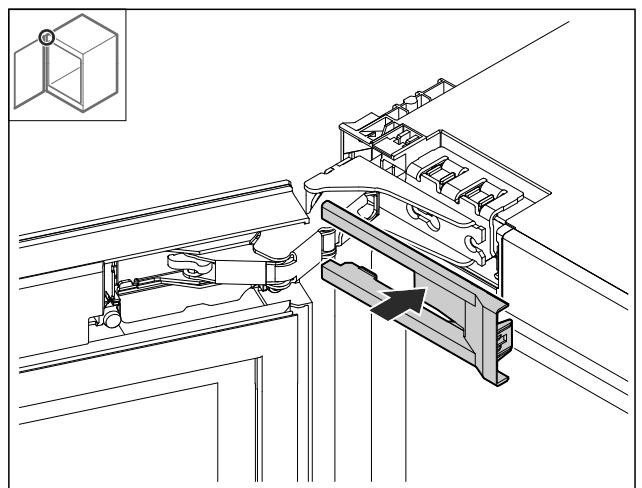
Fig. 28 ► Abdeckung aufsetzen.
