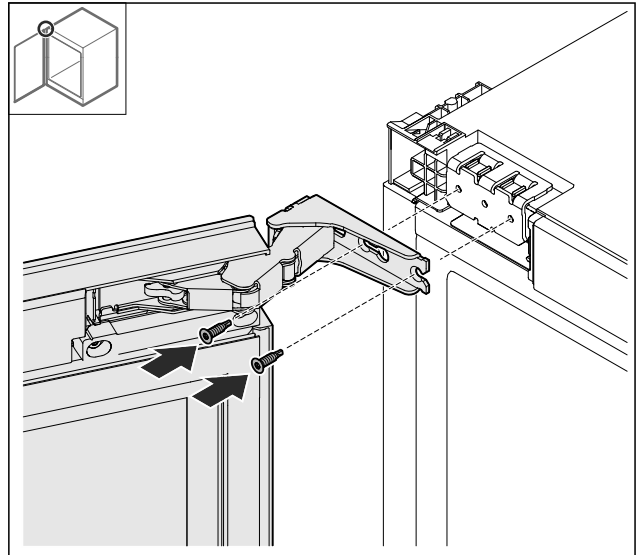
Fig. 26 ► Tür oben anschrauben.
