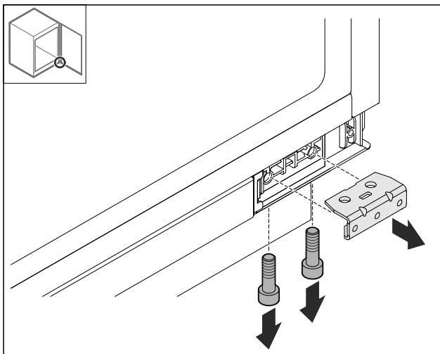
Fig. 24 ► Winkel demontieren.
