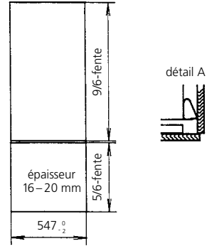
panneaux de porte EU
