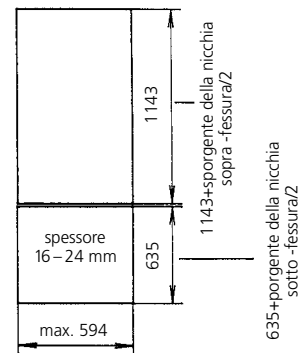
panello della porta EU
