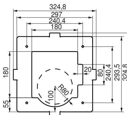
Boorsjabloon (aanzicht X)
