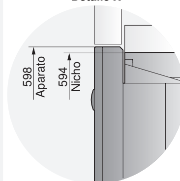
Detalle X
