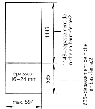
panneaux de porte EU
