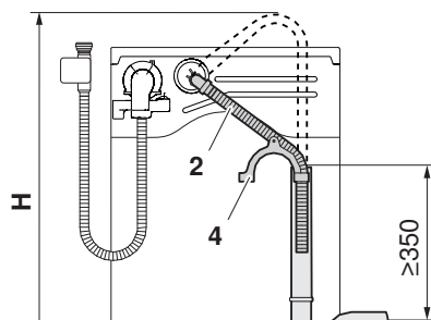
Scarico nel tubo verticale
