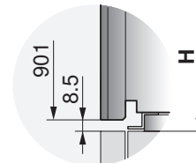
Detail Y
