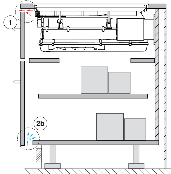
无扁平通道系统的空气循环模式
