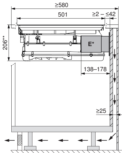
无导向空气循环模式, 带伸缩接头 (E*)
