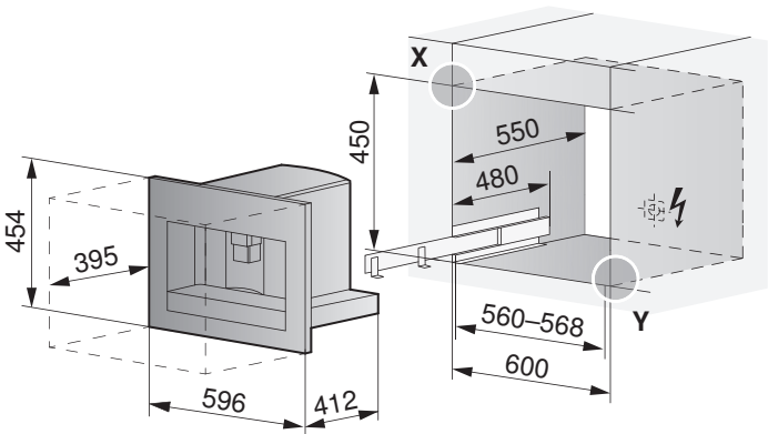
设备前部尺寸：细节图 X/Y (参见页码 9)
