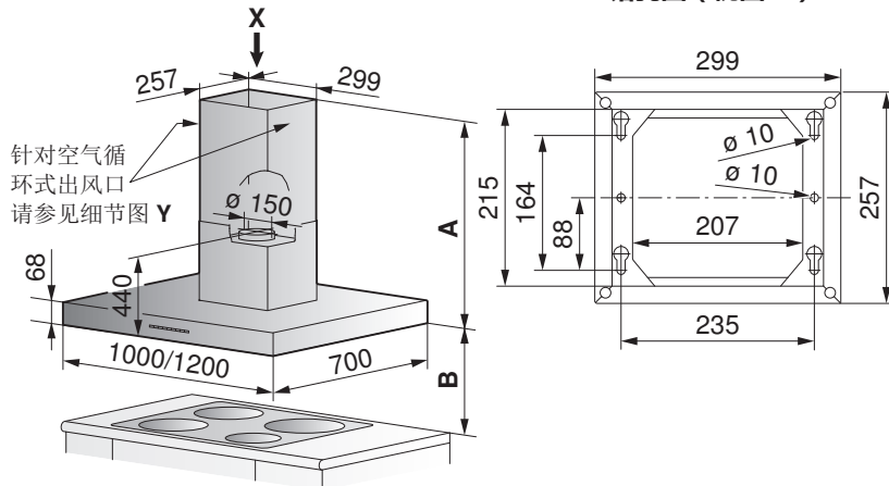
钻孔图 ( 视图 X )
