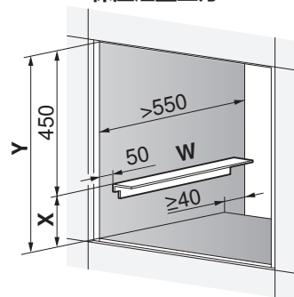
保温层上方
