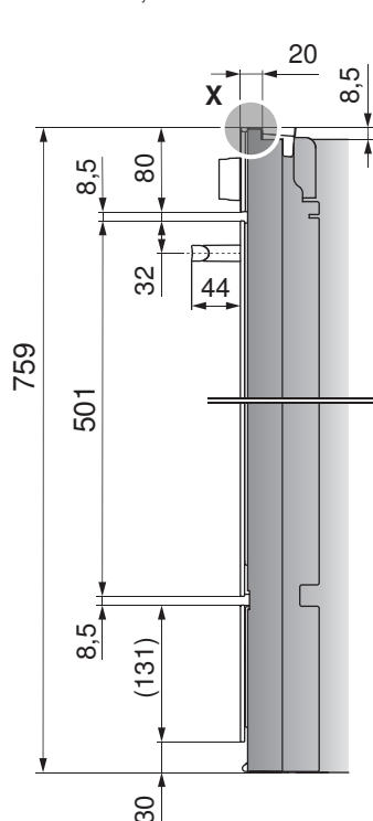
Four, dans armoire haute
