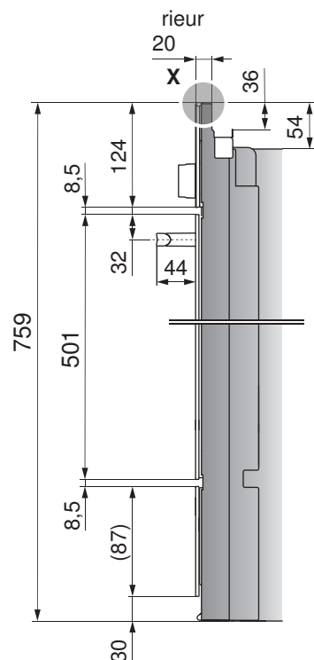
Four/cuisinière dans élément infé- rieur
