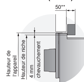
Détail X (EURO)
