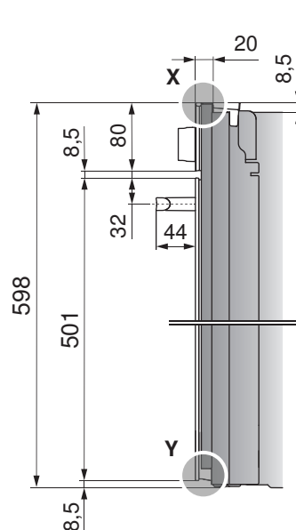
Four/cuisinière sans tiroir
