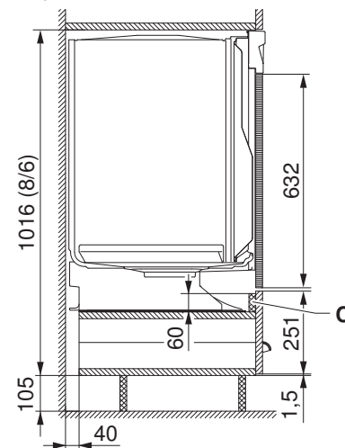
Coupe d'une variante d'encastrement
